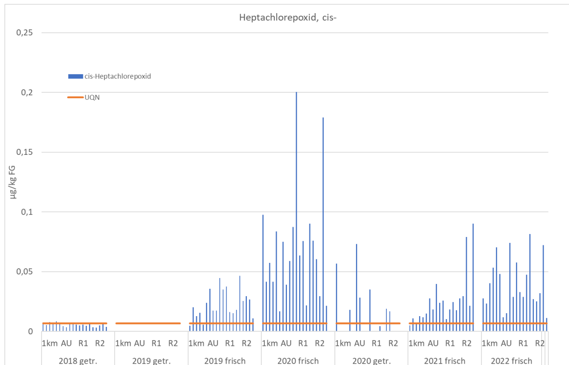
Abbildung 4-106 Gehalte von cis-Heptachlorepoxid im Klieschenmuskel 2018-2022 gemessen an gefriergetrocknetem und/oder frischem Material (Bezugsbasis: Frischgewicht)
