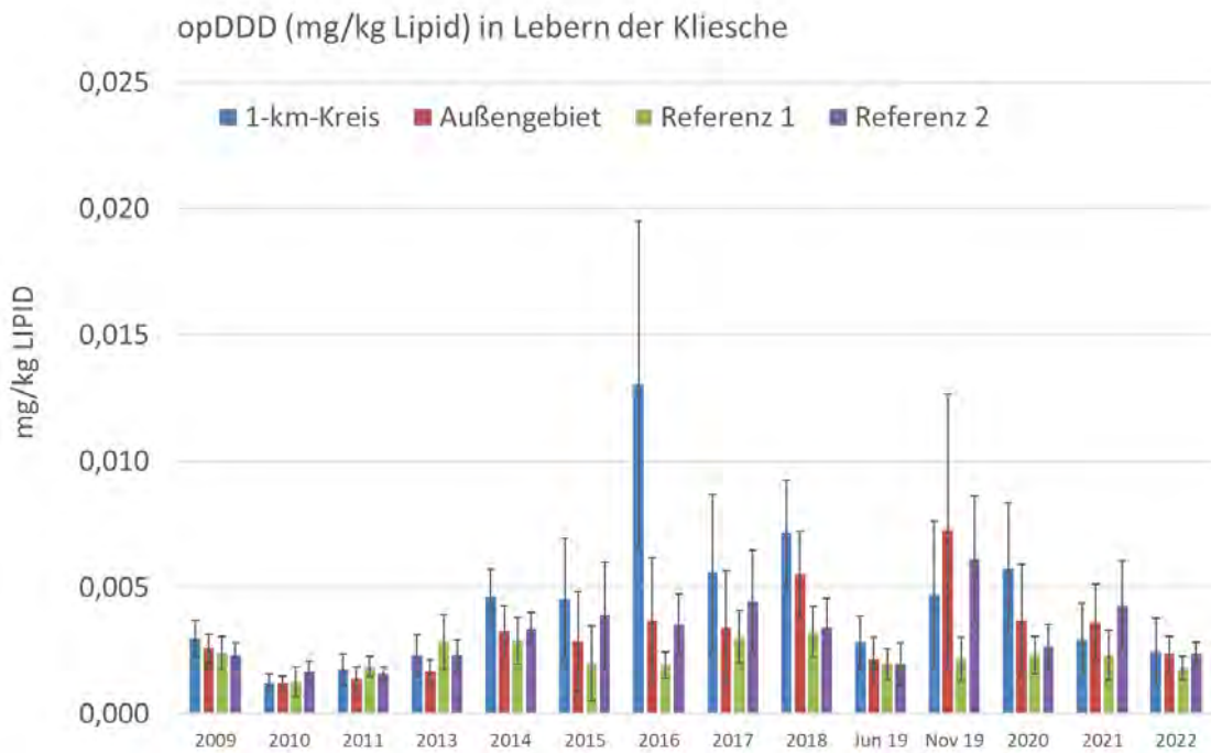
Abbildung 4-79 Mittlere Gehalte an op-DDD im Lebergewebe der Kliesche (Bezugsbasis Lipid)
