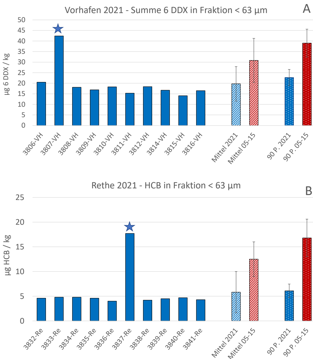
Abbildung 3-5 Einzelwerte der Freigaben aus dem Vorhafen 2021 (Summe 6DDX, A) und Rethel 2021 (HCB, B) in Relation zu den Mittelwerten und dem 90. Perzentil der jeweiligen
