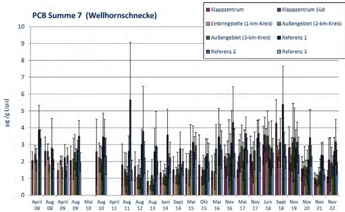
Abbildung 4-54 Belastung der Wellhornschncken: Summe der 7 PCB Kongenere von 2008 bis 2022 (Bezugsbasis Lipid)
