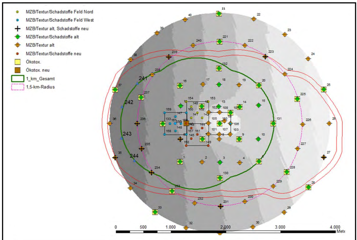
Abbildung 4-7 Stationsnetz im Nahbereich der Verbringstelle (2-km-Kreis) im Jahr 2021 und 2022 (Der rosafarbene Kreis (1,5-km-Radius) mit der Ausbuchtung in grün im Westen mit den Stationen 241-244 stellt den Einbringbereich dar, s. Text im Kasten am Anfang des Kapitels)
